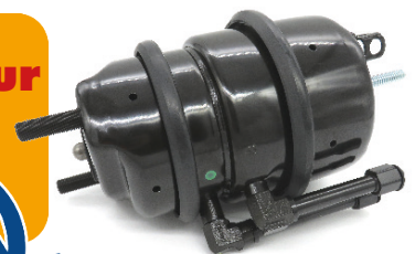
4192016 CYLINDRE DE FREIN TYPE 16/24 SAF
