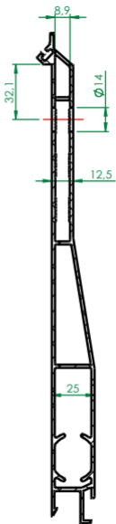
B-B (1 : 2)
