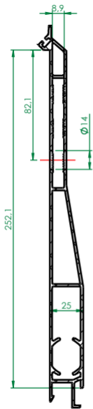
A-A (1 : 2)
